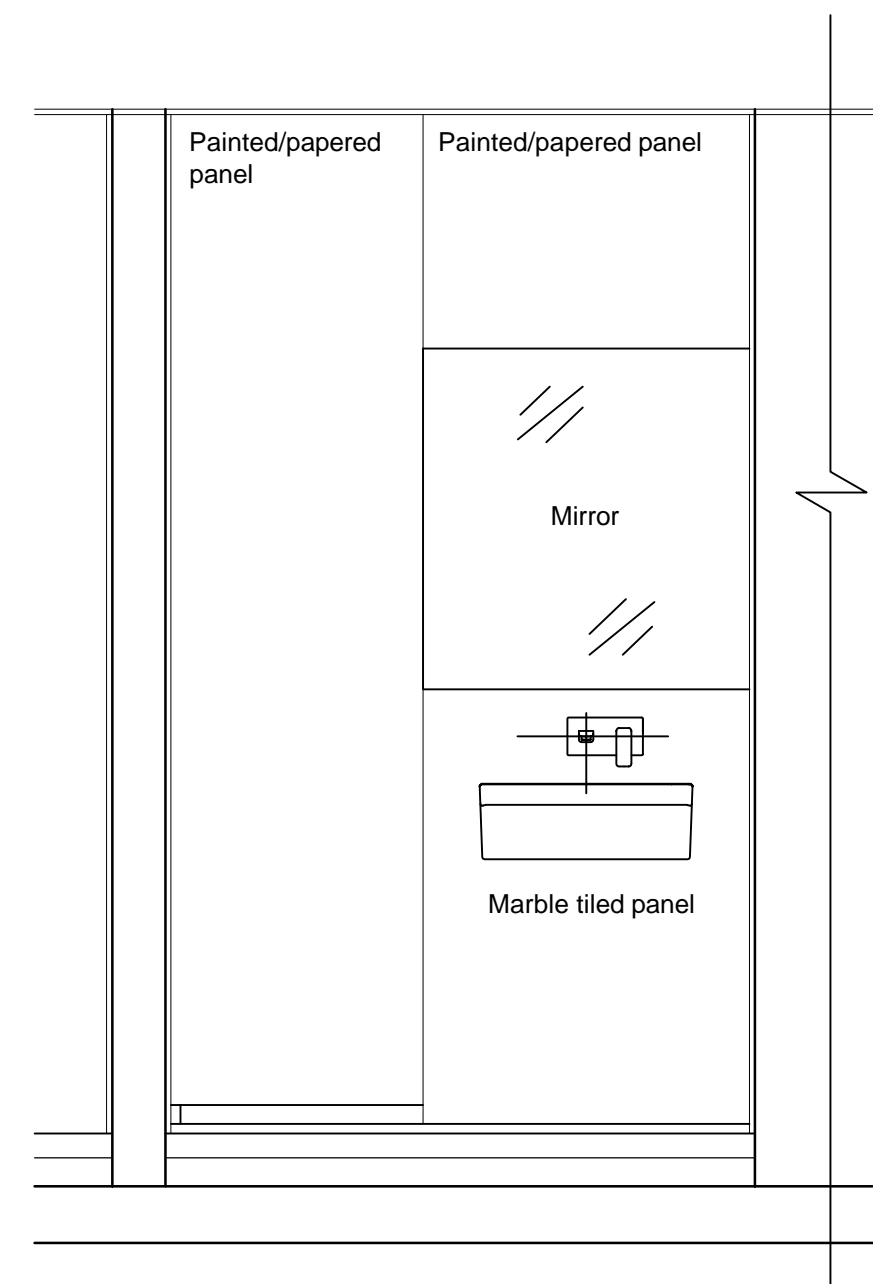
Elevation B
