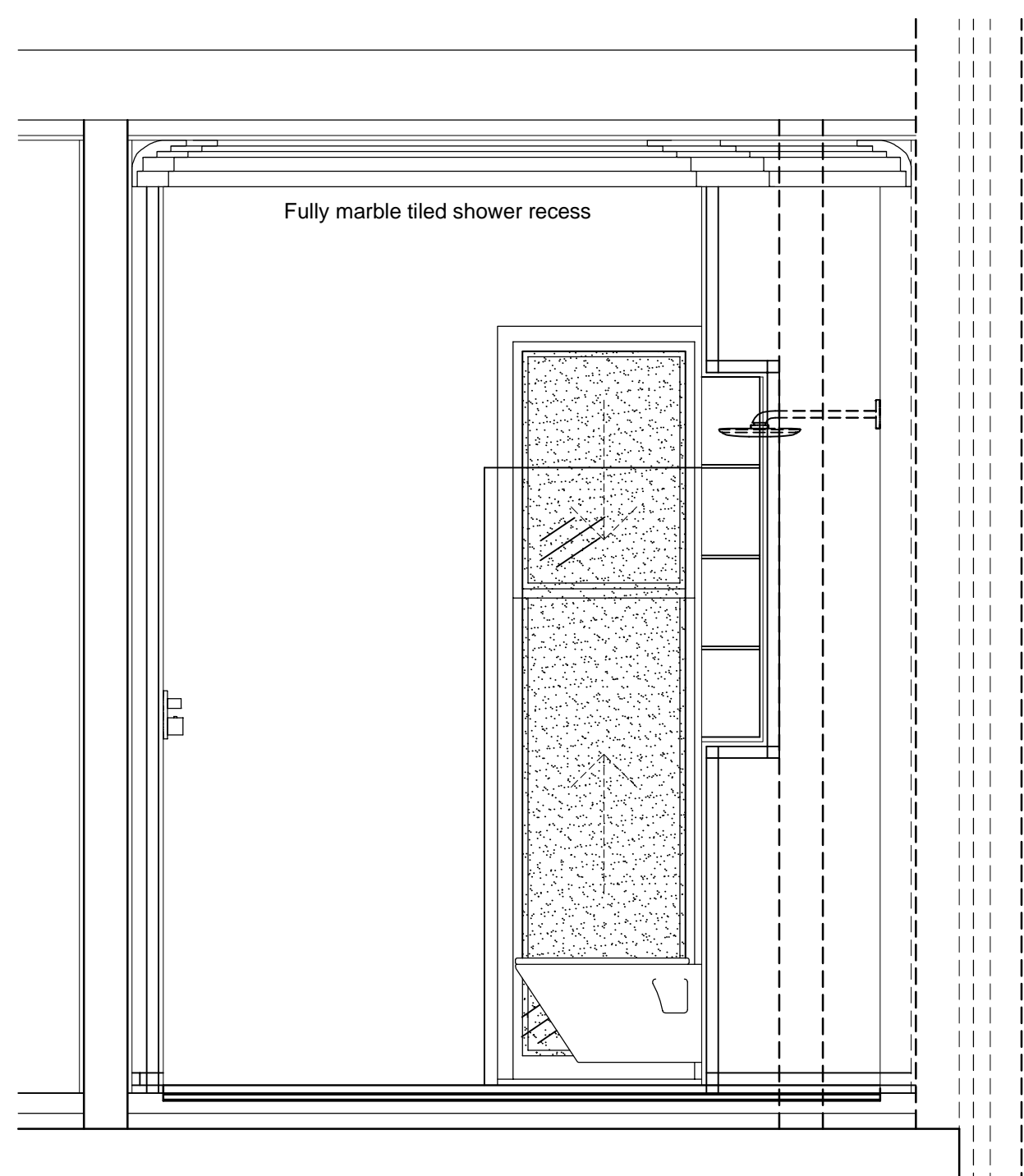
Elevation A
