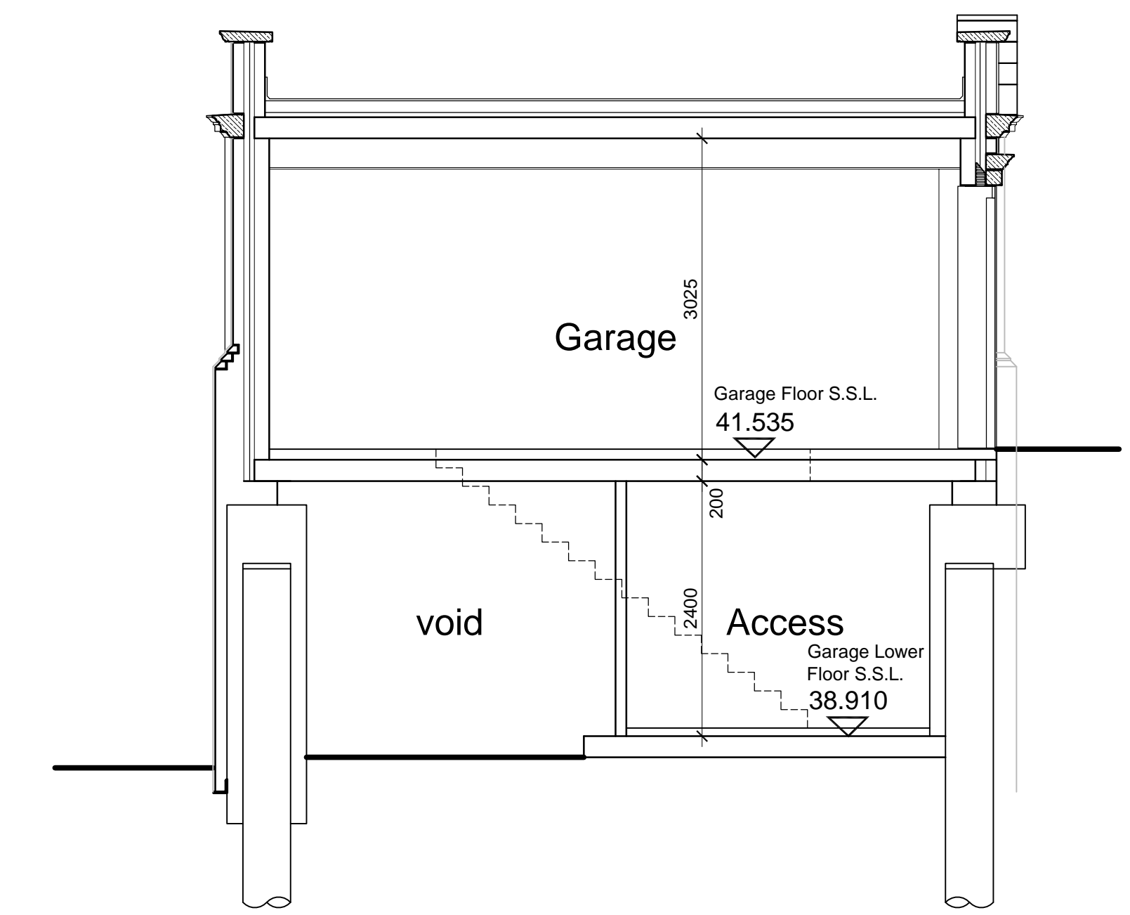
Section E - E
